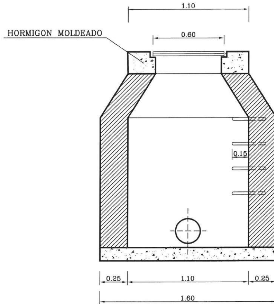
ALZADO-SECCION
